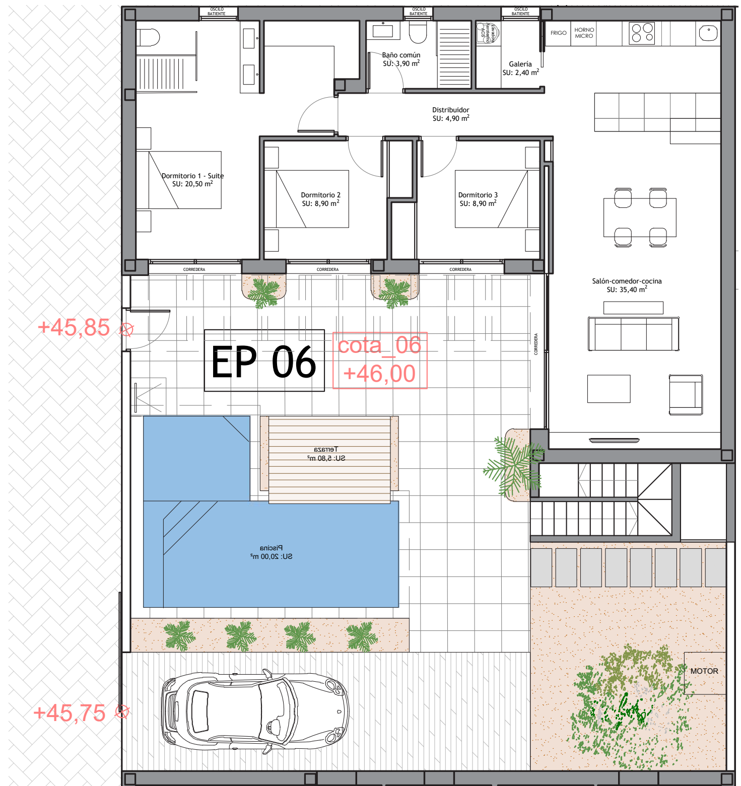
PLANTA BAJA
