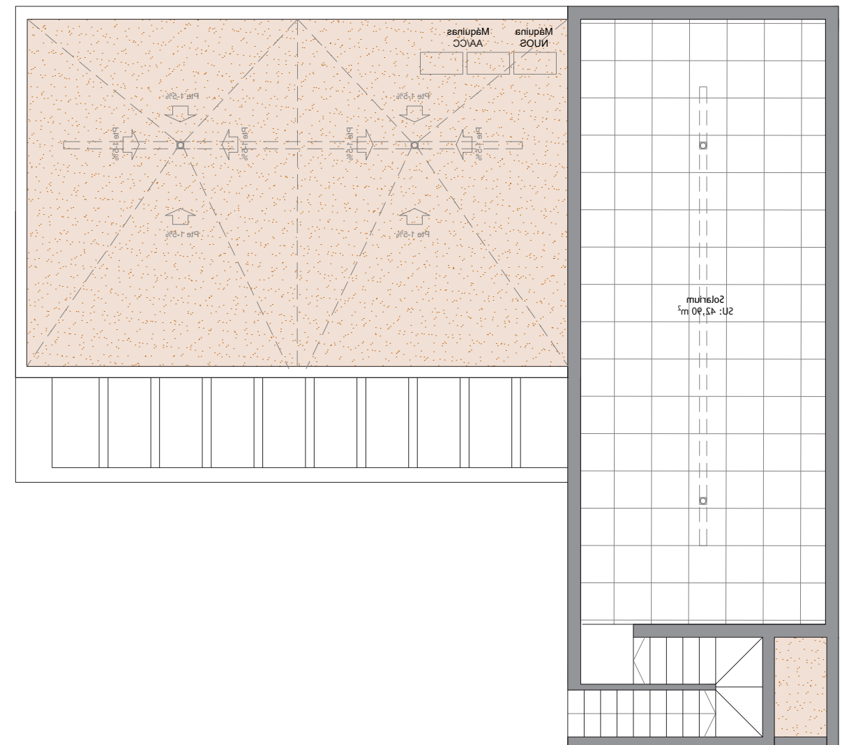
PLANTA SOLARIUM
