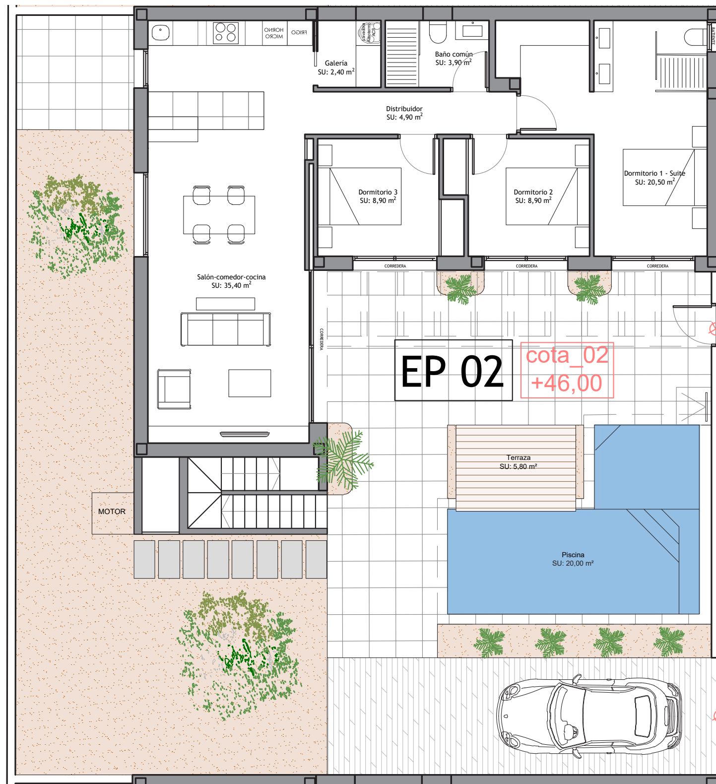
PLANTA BAJA
