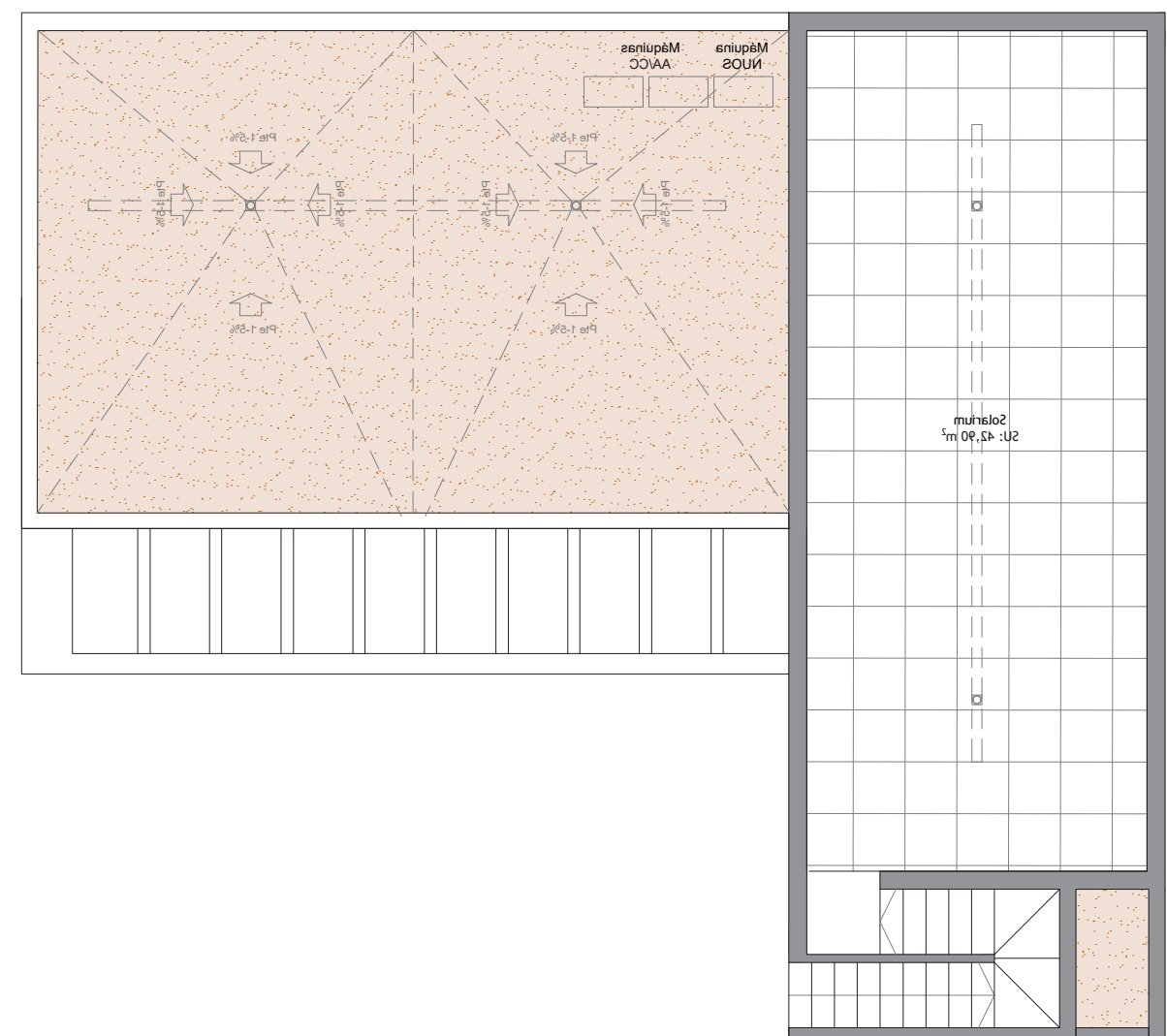
PLANTA SOLARIUM
